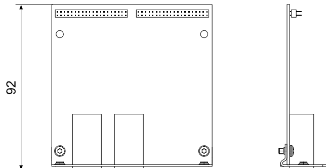
Fig. 2: Dimensions
